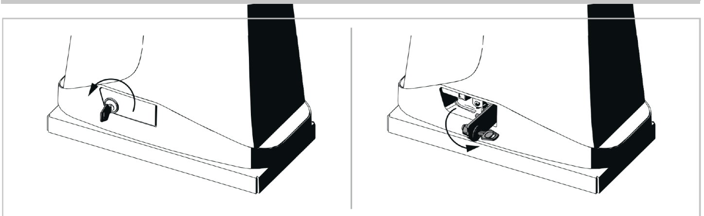
Fig. 8 - Χειροκίνητη απασφάλιση έκτακτης ανάγκης
