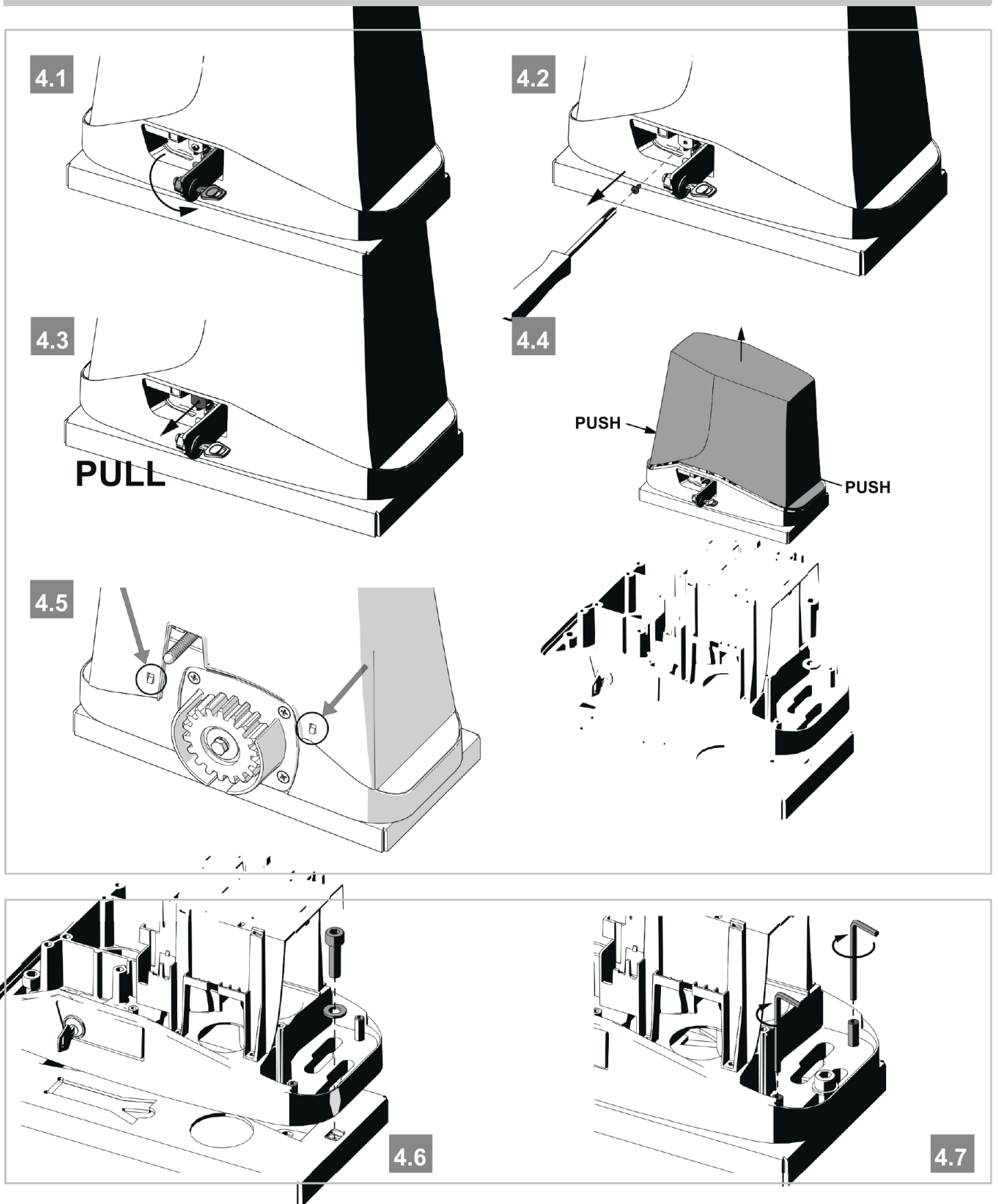
Fig. 4 - Στερέωση
