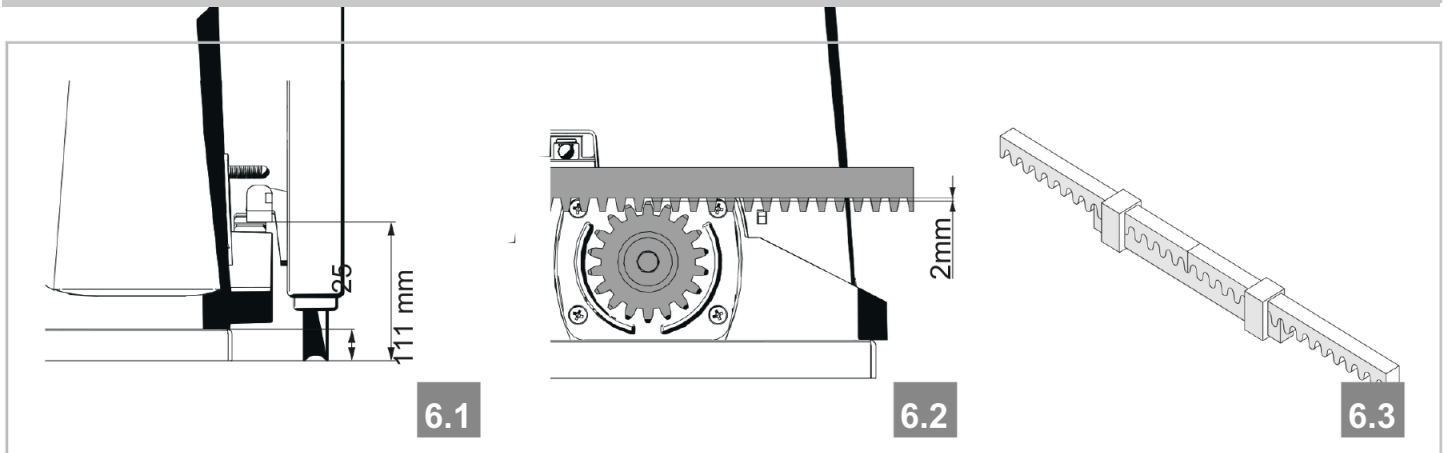
Fig. 6 - Στερέωση κρεμαγιέρας
