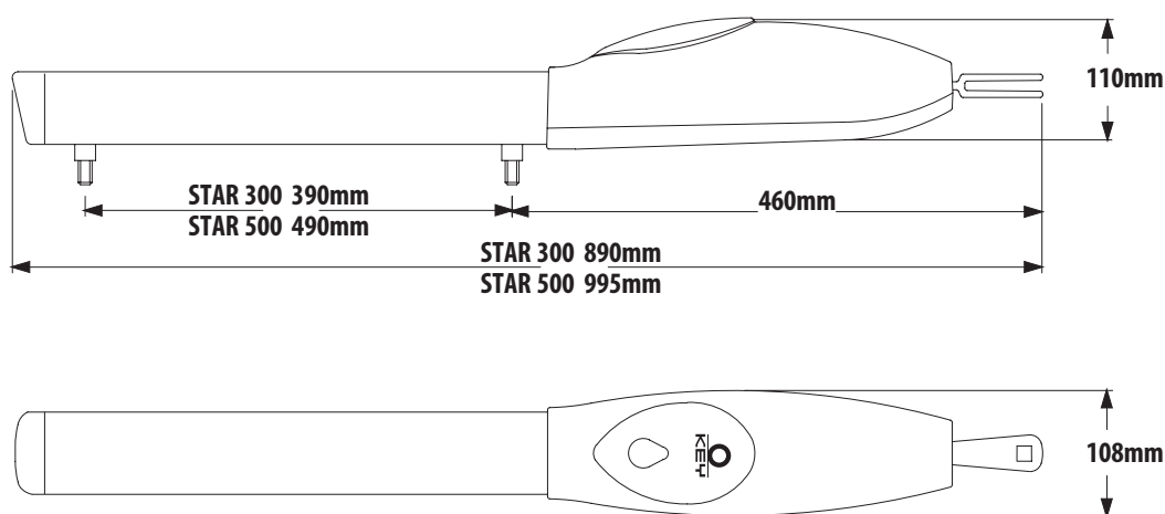
Fig. 1 IT - Dimensioni d'ingombro EN - Space dimensions DE - Abmessungen ES - Dimensiones
